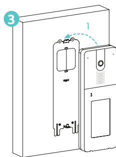
3 AGGANCIARE PARTE SUPERIORE HOOK THE TOP
