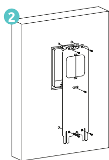
2 FISSAGGIO PIASTRA FIX METAL PLATE
